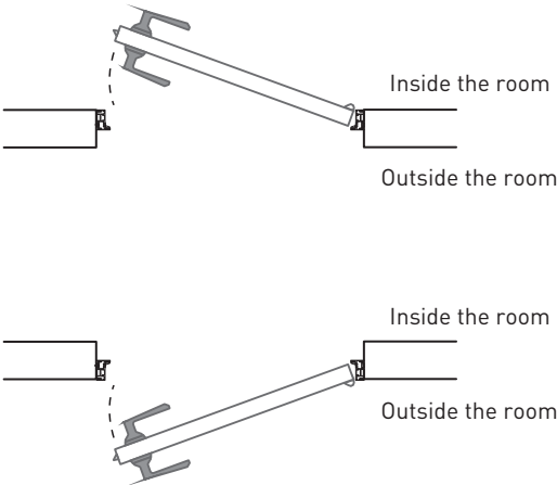
FLAT JAMB
